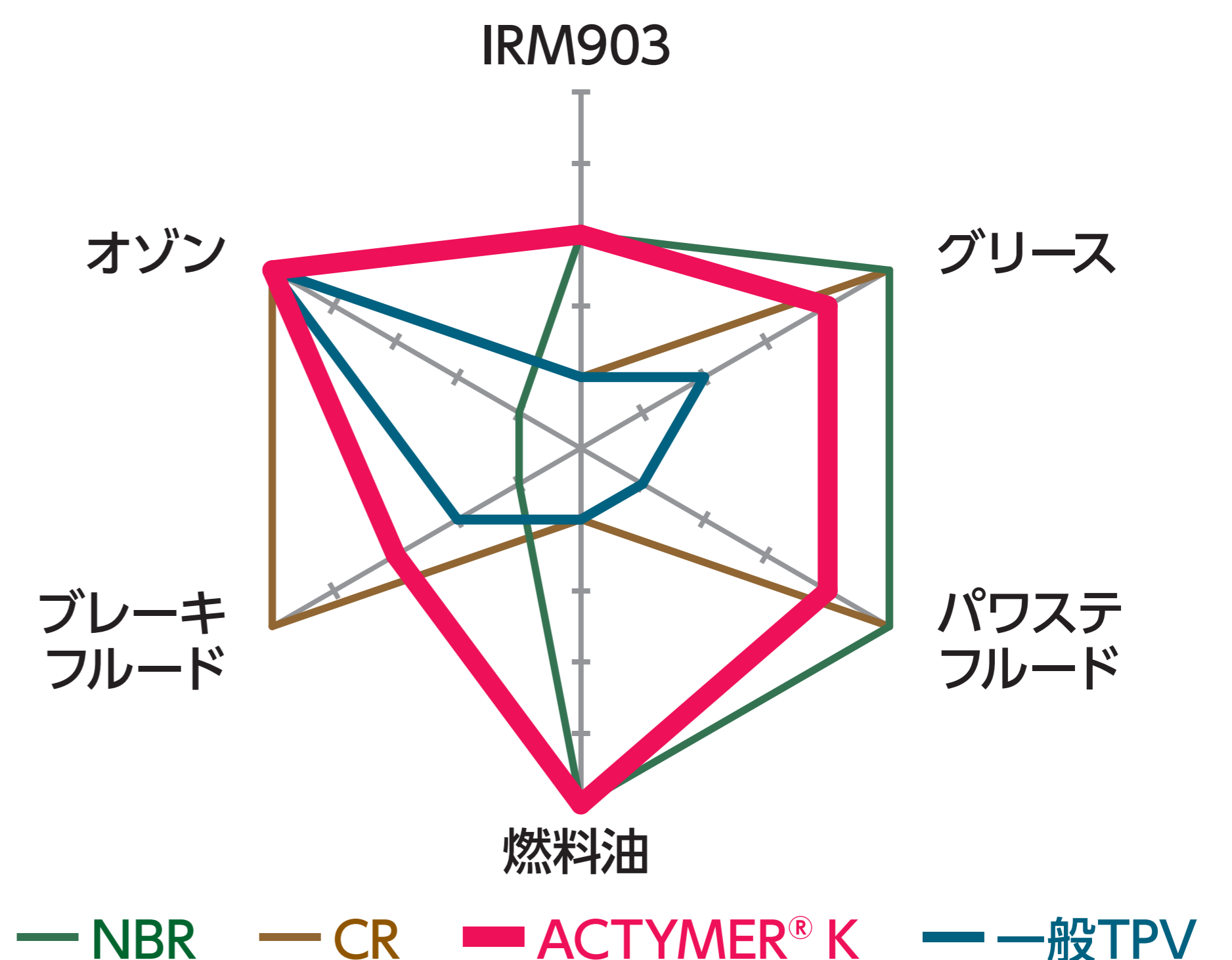
NBR/CRゴムと各種オイル及びオゾンへの耐久性比較
