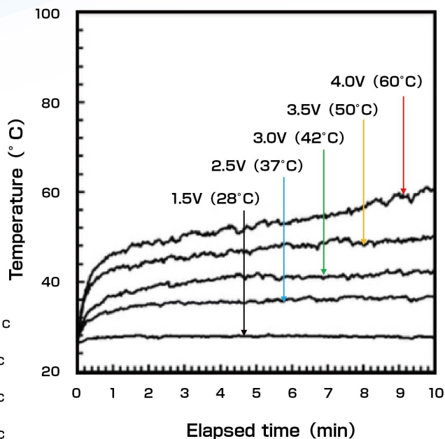
電圧印加時間と薄膜表面温度の関係
