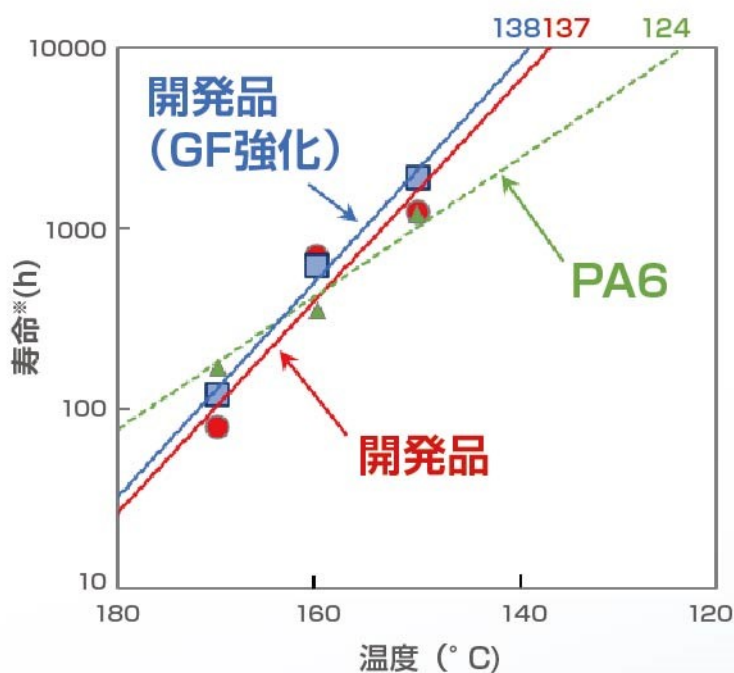
＜PA6と比較したアレニウスプロット＞
